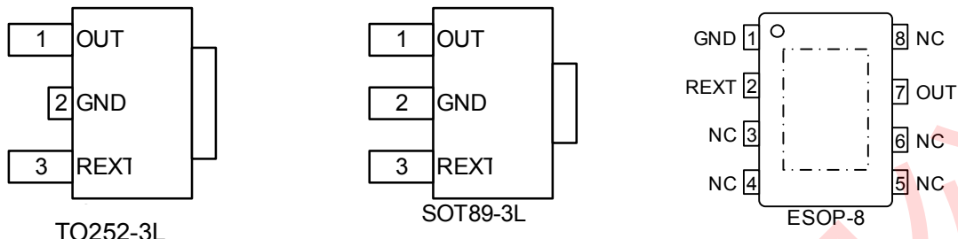
图 2. PT4515NF 管脚定义图
