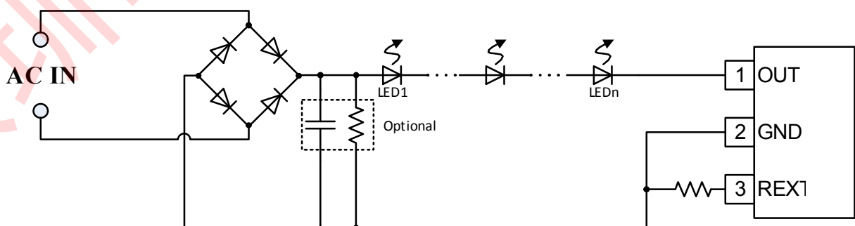
图 1. PT4515NF 典型应用电路图
