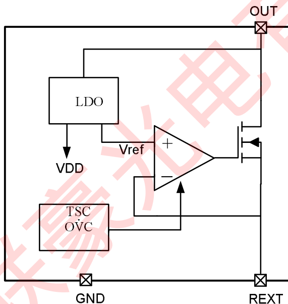
图 3. PT4515NF 内部模块简化图
