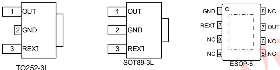
图 2. PT4515NH 管脚定义图
