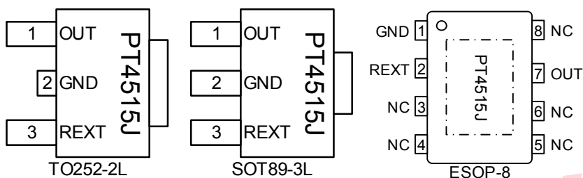
图 2. PT4515J 管脚定义图
