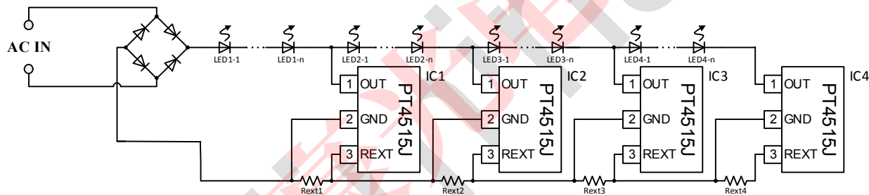
图 5. PT4515J 串联应用电路原理图
