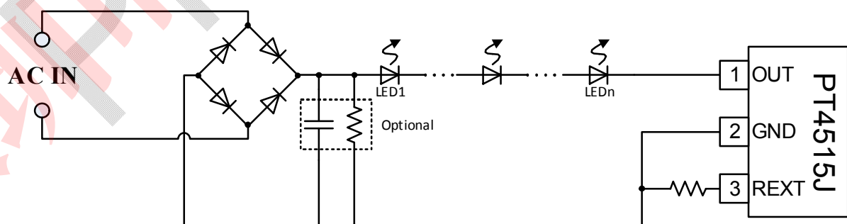
图 1. PT4515J 典型应用电路图
