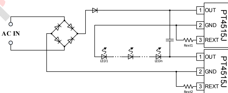
图 7. PT4515J 填谷电路应用电路原理图 2
