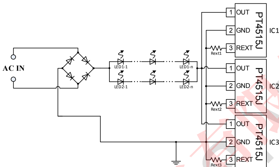
图 4. PT4515J 并联应用电路原理图
